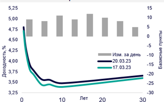
Кривая UST
