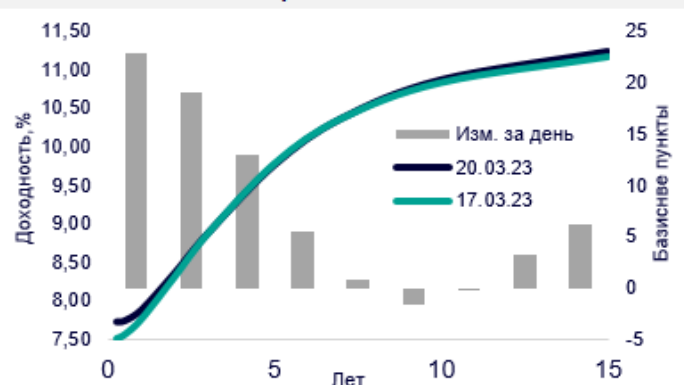
Кривая ОФЗ
