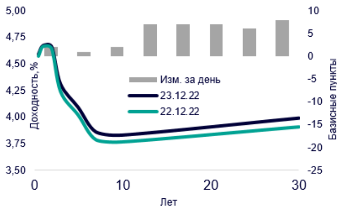
Кривая ОФЗ
