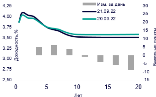
Кривая ОФЗ
