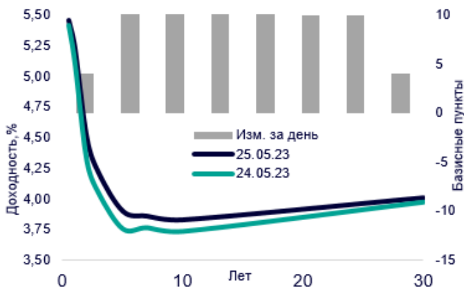
Кривая ОФЗ
