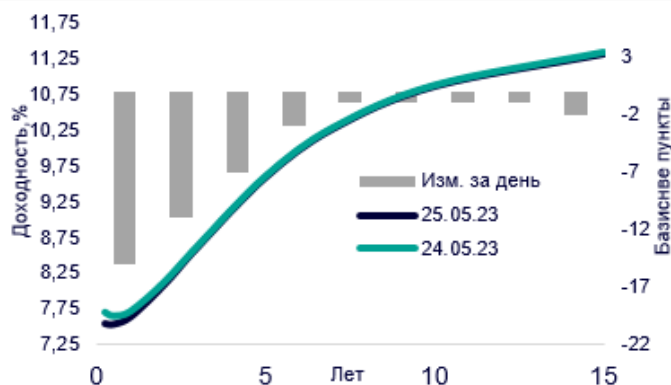
Кривая ОФЗ
